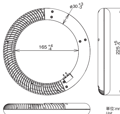
外形寸法図
