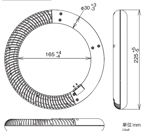
外形寸法図
