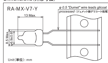
Dimensions (外形寸法)
