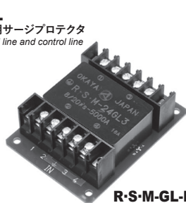
R-S-M-GL-PT データ通信用サージプロテクタ For data signal line and control line
