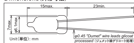
Dimensions (外形寸法)
