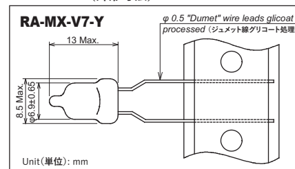
Dimensions (外形寸法)
