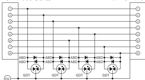
モジュージャック (RJ45)
