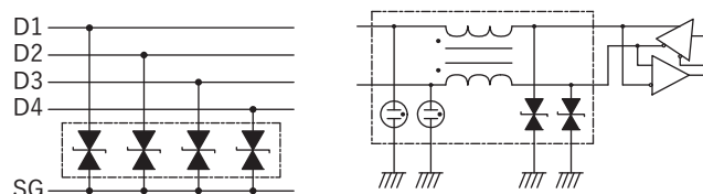
e) データライン保護(アラートタイプ)
