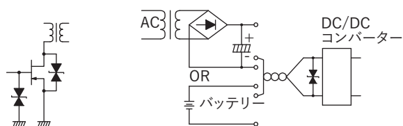
a) スwitchingサージ保護
