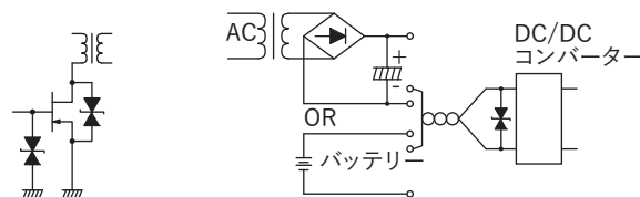
a) スイッチングサージ保護
