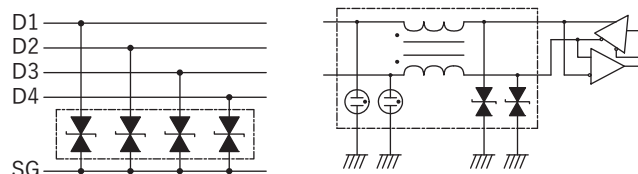
e) データライン保護(アレータイプ)
