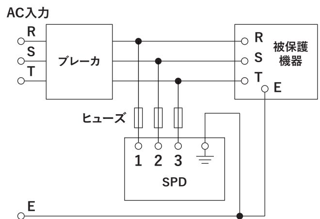
(図-B) 三相交流回路での使用例
